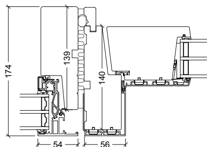
Med VELFAC Ribo inåtgående dörr. Husk täckplåt*.
