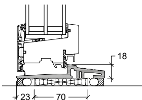
Fönsterdörr
