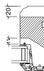
VELFAC Classic + Ribo fast utan bäge, 2-glas kassett
