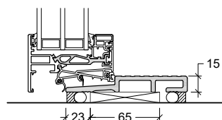
Fönsterdörr
