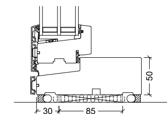
Fönster och fönsterdörr
