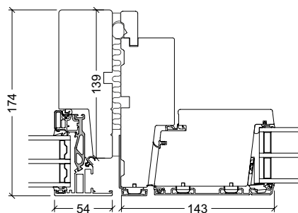
Med VELFAC Ribo utåtgående dörr. Husk täckplåt*.
