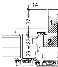
123mm karm
