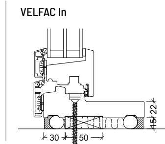
Fönsterdörr
