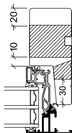
VELFAC 200 + Edge
