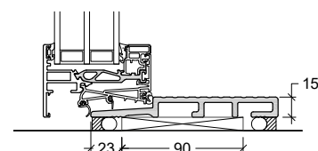
Fönsterdörr
