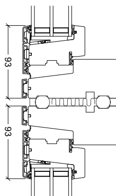
Vertikal sammanställning fönster med fönster
