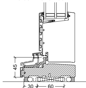
Ytterdörr/Terrassdörr
