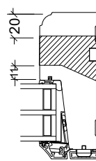
VELFAC Classic + Ribo fast utan bäge, 3-glas kassett
