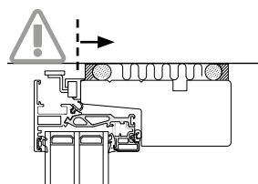
VELFAC 200 skjutdörr Foga enbart från den streckade linjen
