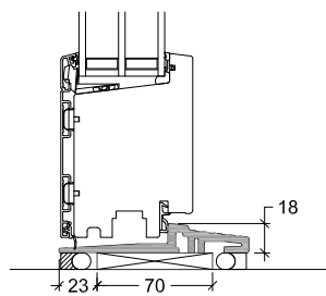
Ytterdörr/Terrassdörr
